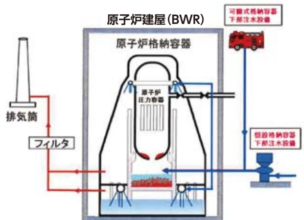
図3. 格納容器破損防止対策
