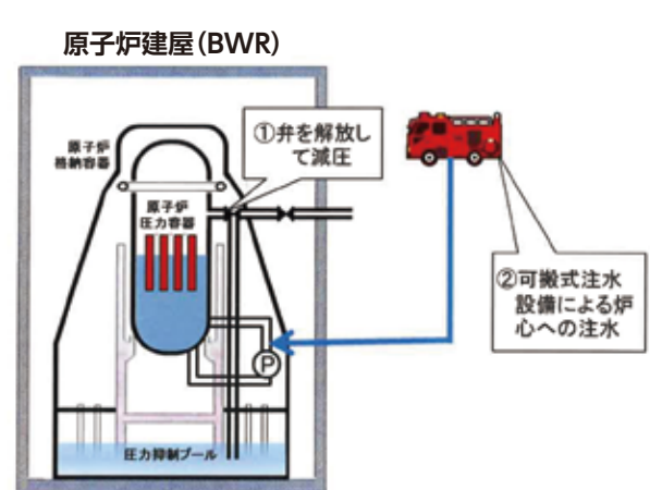
図2. 炉心損傷防止対策
