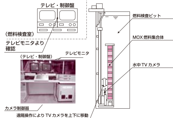
MOX輸入燃料体の外観確認検査の方法
