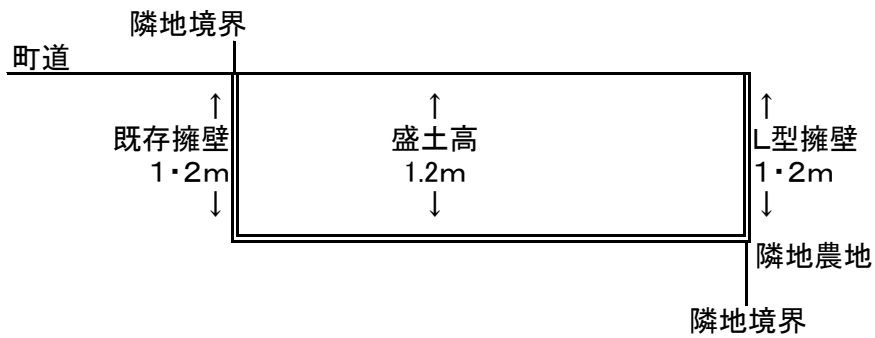
断面図
