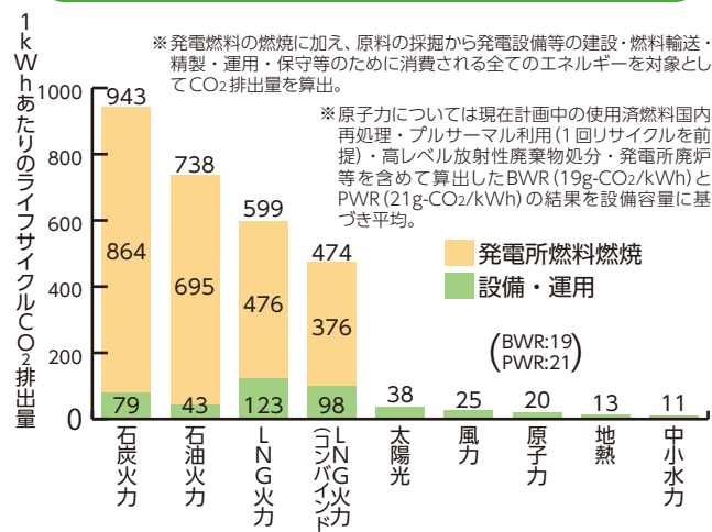
各種電源別のライフサイクルCO 2 排出量
